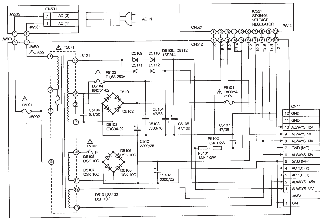
Принципиальная схема источника питания видеомэагнитофона VHR-220EE фирмы SANYO
